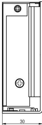
右视图
