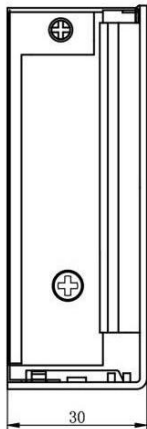
右视图
